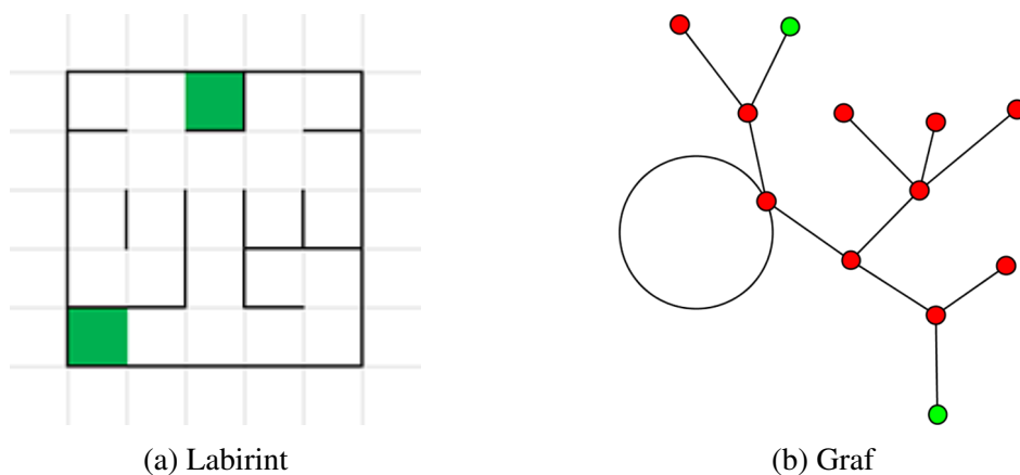
Slika 3.2: Reprerentacija labirinta grafom
