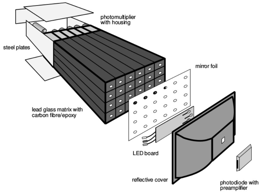
Slika 2.7: Shematski prikaz jednog supermodula PbI 2 detektora, sastavljenog od 6 × 4 modula. Preuzeto iz [13].
