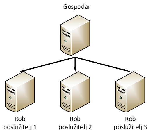
Slika 2.3 Gospodar-rob arhitektura
