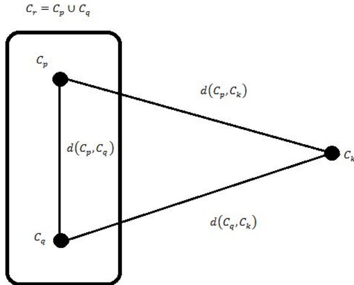
Slika 1.2: Tri klastera
