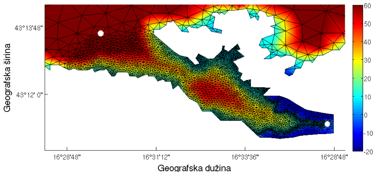
Slika 4.10: Isječak iz mreže modela za područje Zaljeva Stari Grad. Osim batimetrije u mrežu je uključena topografija (m). Bijele točke označavaju lokacije čvorova na ulazu i vrhu zaljeva koje su korištene za prikaz vremenskih nizova na slikama 4.11 i 4.12.
