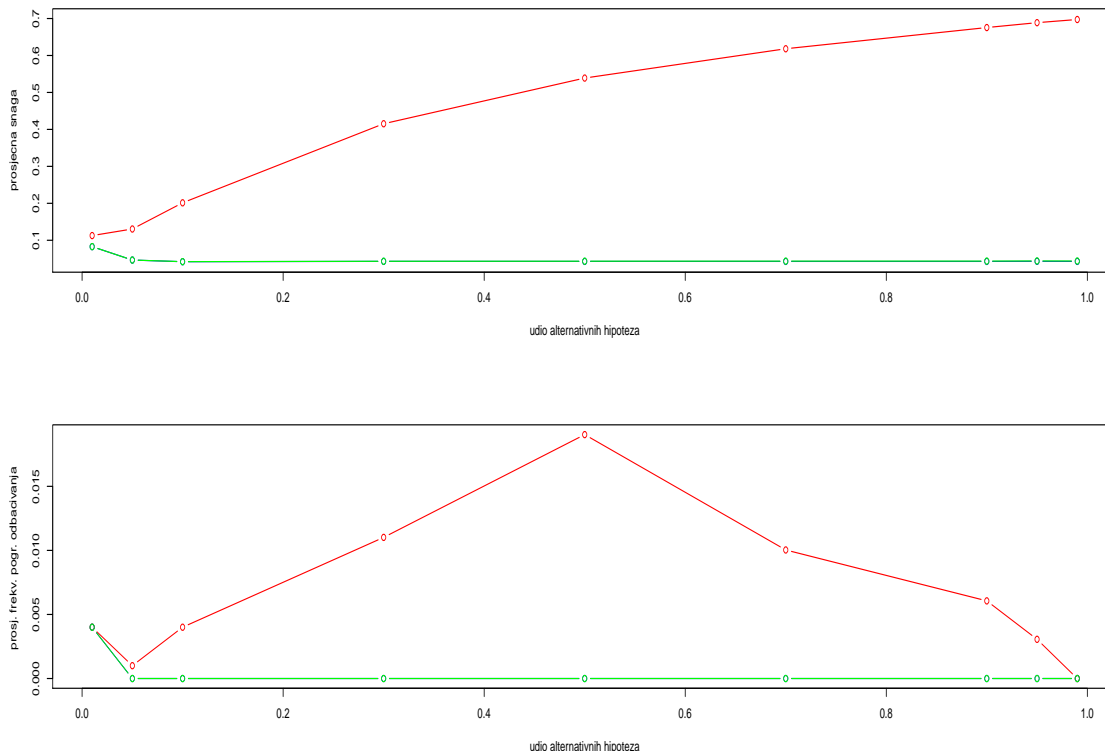
Slika 3.3: prosječna snaga i prosječna frekvencija pogrešno odbacjenih nul hipoteza za q^* = 0.1 , odnosno \alpha = 0.1 (crvena linija ↔ FDR, zelena linija ↔ Holm's i FWER)
