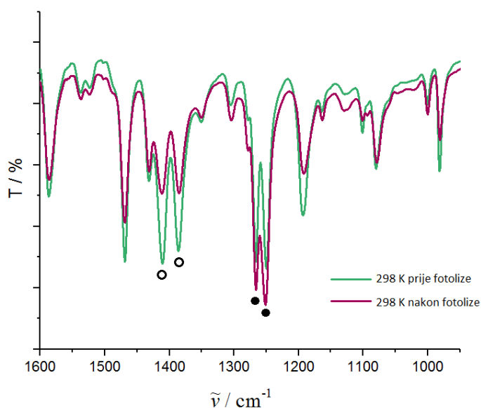
Slika 26. Usporedba IR spektara spoja 1 snimljenih pri sobnoj temperaturi nakon sublimacije i prije fotolize (zeleni spektar) te nakon fotolize (crveni spektar). Vrpce istezanja Z-azodioksidne veze označene su šupljim crnim kružićem ( \circ ), dok su vrpce istezanja E-azodioksidne veze označene punim crnim kružićem ( \bullet )
