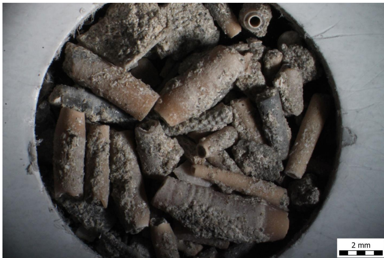
Slika 7. Najčešći fosili iz uzorka broj 3, izdvojeni tehnikom muljenja (mokrog prosijavanja)
