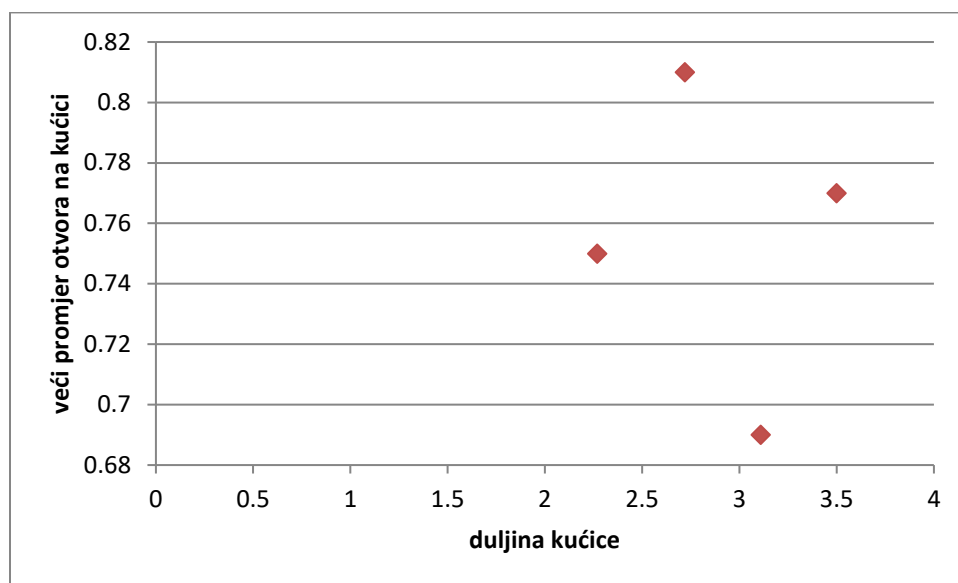
Slika 19. Odnos duljine kućice i većeg promjera dentaliuma
