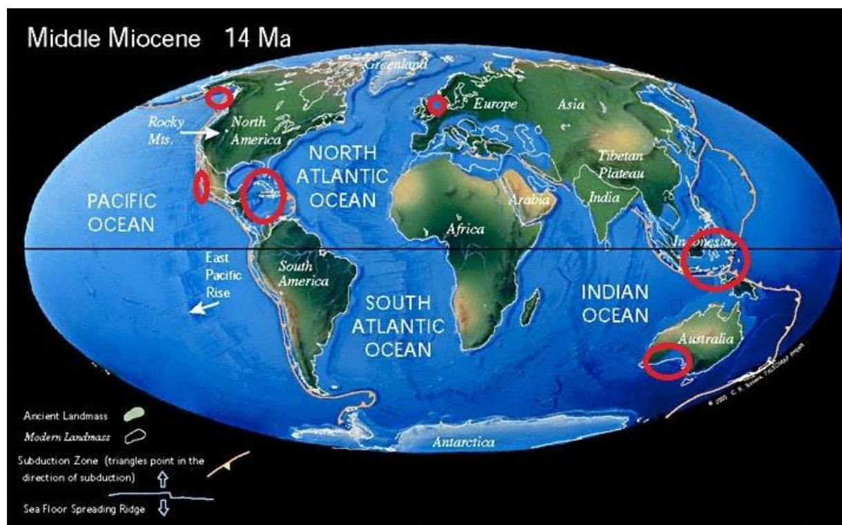
Slika 40. Zastupljenost roda Cadulus u svijetu za vrijeme miocena (paleogeografska rekonstrukcija prema www.scotese.com )
