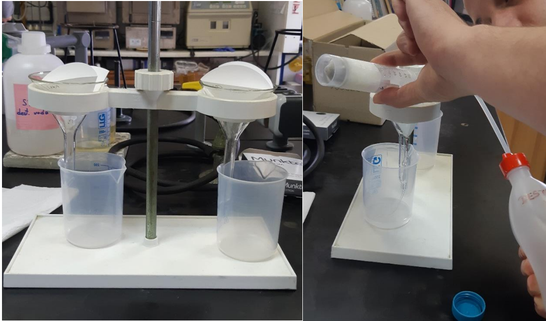
Slika 3.11. Prikaz aparature te postupka izdvajanja lake frakcije
