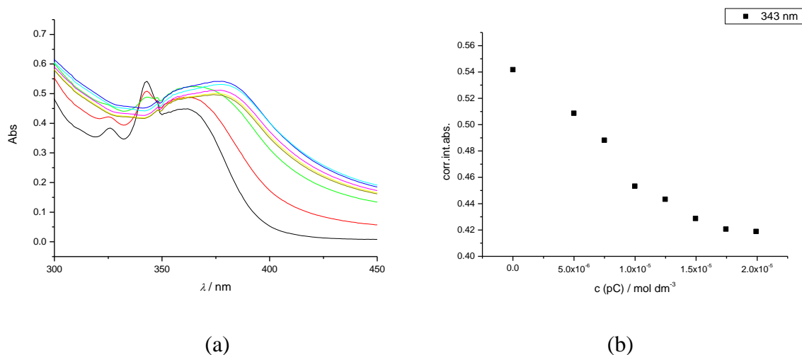
Slika D6. (a) Promjene u UV/Vis spektru SG224 prikome titracije s pC; (b) Pad apsorpcije spoja SG224 pri valnoj duljini maksimalne apsorpcije, \lambda_{\max} = 343 nm, prilikom titracije spoja s pC (kakodilatni pufer, pH 7).
