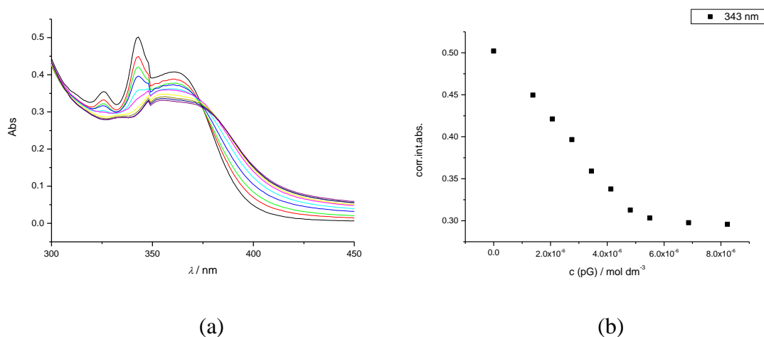
Slika D5. (a) Promjene u UV/Vis spektru SG224 prikome titracije s pG; (b) Pad apsorpcije spoja SG224 pri valnoj duljini maksimalne apsorpcije, \lambda_{\max} = 343 nm, prilikom titracije spoja s pG (kakodilatni pufer, pH 7).
