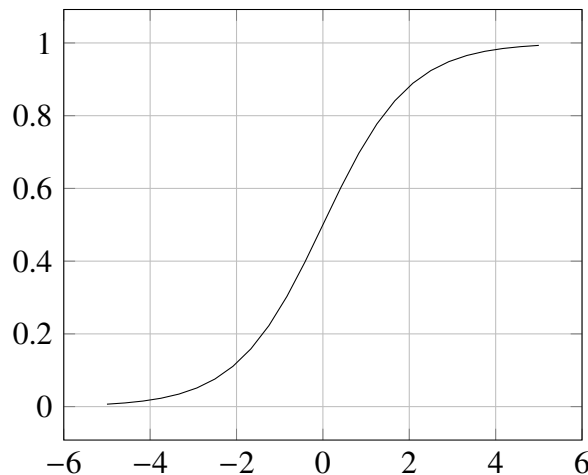
Slika 1.1: Logistička funkcija
