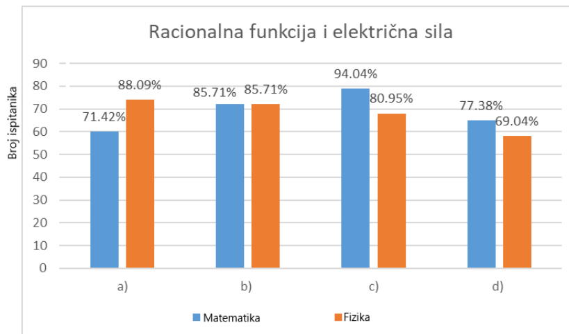
Slika 3.8: Dijagram 2; Prva dva stupca prikazuju rješenost zadatka 2.a) (plavi) i 6.c) (narančasti). Stupci pod b) prikazuju rješenost zadatka 2.b) i 6.a), stupci pod c) prikazuju rješivost 2.c) i 6.c), stupci pod d) prikazuju rješenost 2.d) i 6.d)
