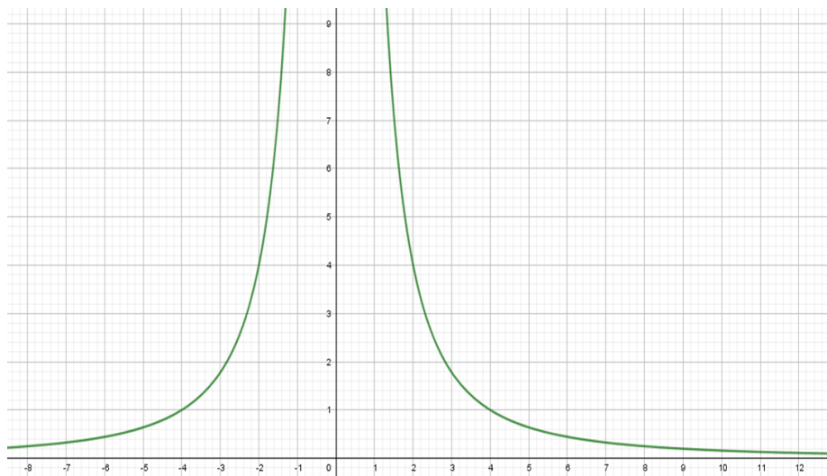
Slika 3.2: graf funkcije
