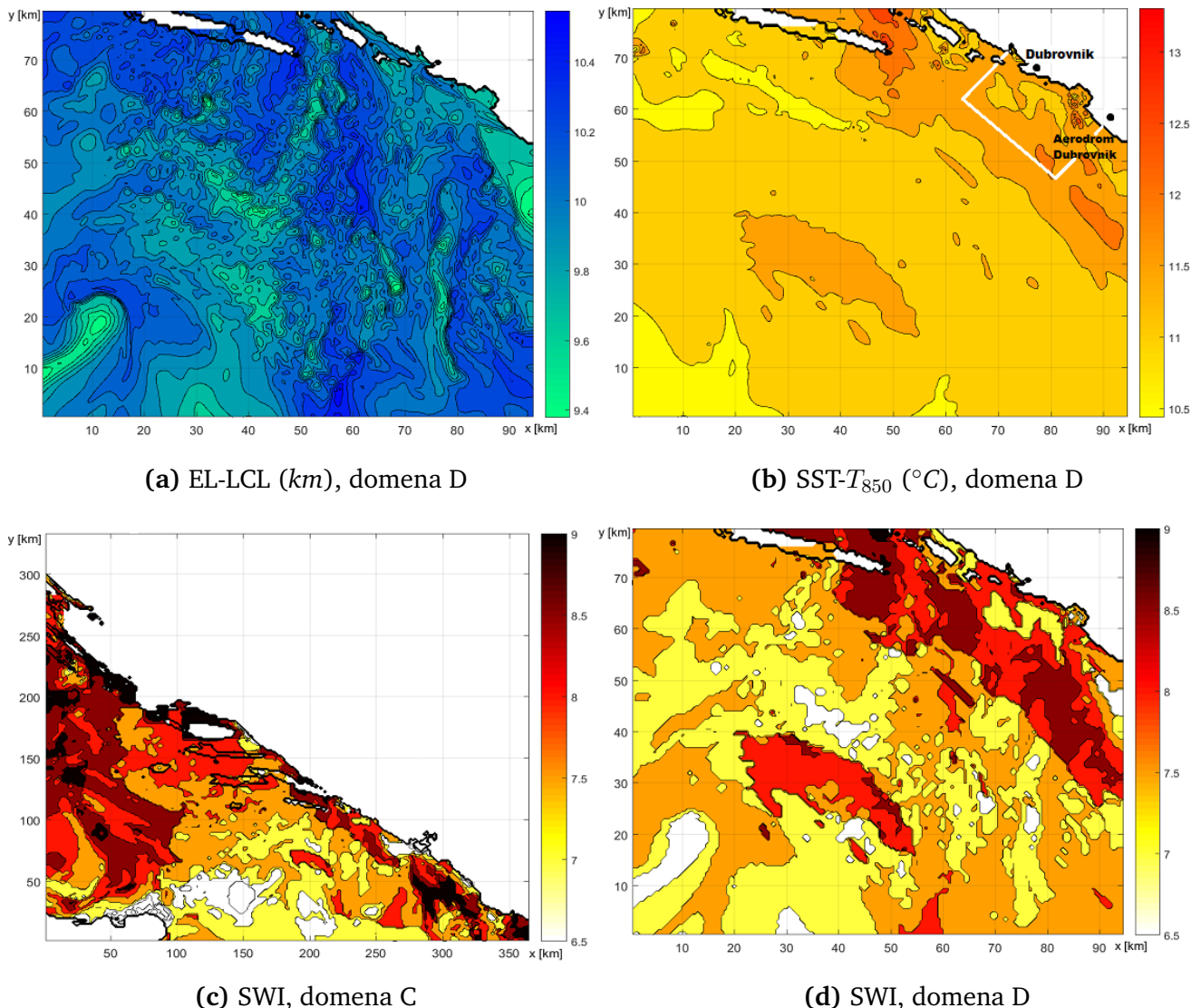
Slika 4.5. Razlike visina EL i LCL, razlike SST i temperature na 850 hPa plohi za domenu D, te vrijednosti SWI za domenu C i D u 07 UTC 28.08.2013. godine.
