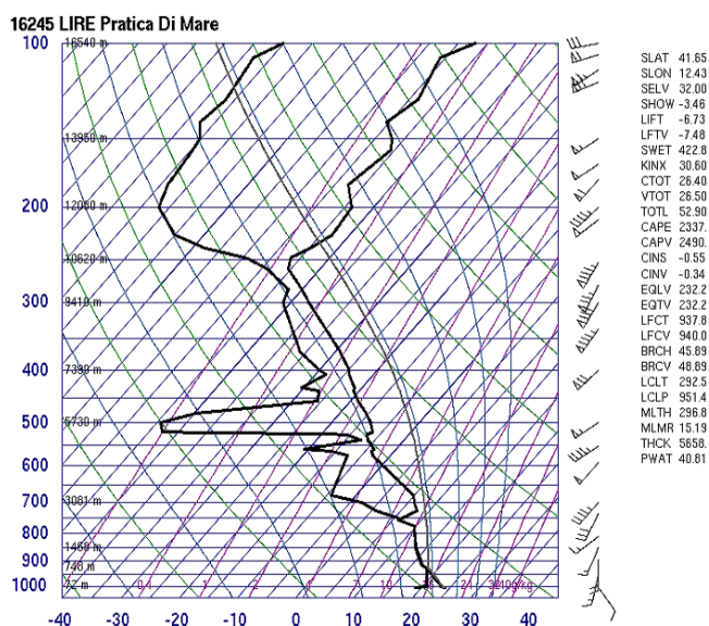
Slika 4.21. Termodinamički dijagram radiosondaže u Rimu u 00 UTC, 30.06.2014. godine (izvor: http://weather.uwyo.edu ).
