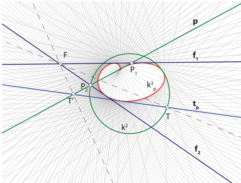
Slika 4.5: Cirkularna krivulja k_p^3 tipa (2,1) dobivena kao nožišna krivulja hiperbole (3c)
