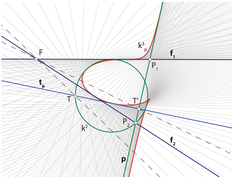
Slika 4.6: Cirkularna krivulja k_p^3 tipa (2,1) dobivena kao nožišna krivulja specijalne hiperbole (3d)
