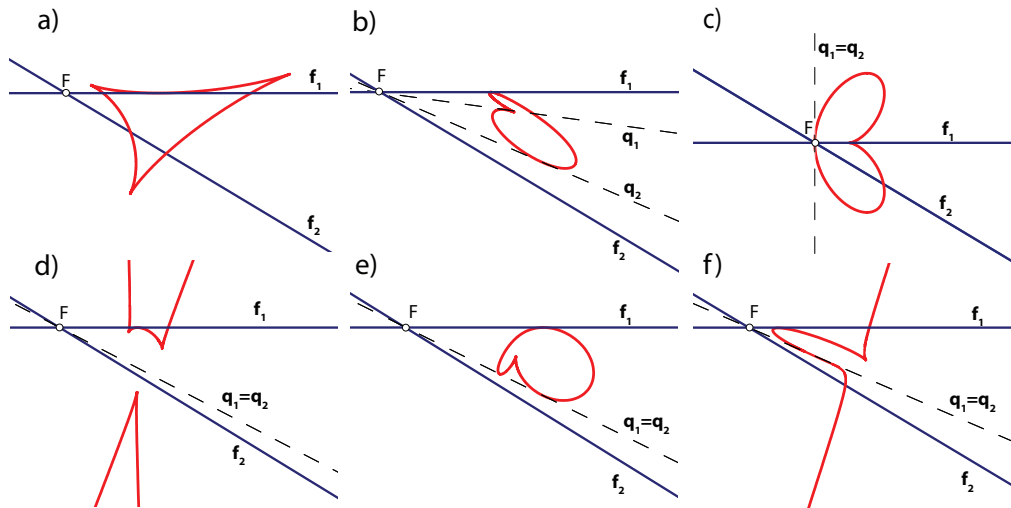
Slika 2.2: Tipovi 1-cikularnih krivulja 3. razreda u \mathbb{QH}_2(\mathbb{R})
