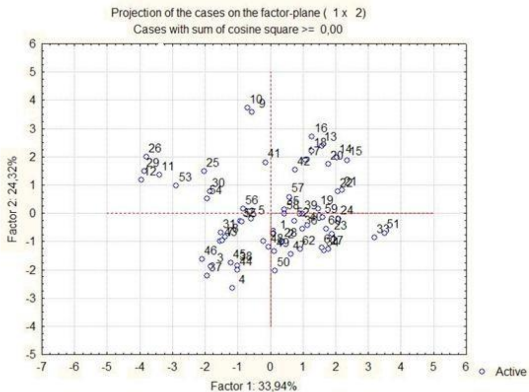
Slika 20. Dijagram faktorskog prikaza za uzorke vina.
