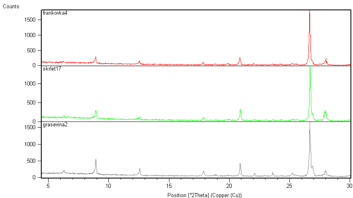
Slika 14. Rendgenogrami za uzorke tla iz vinograda Blagaj za sortu frankovka (crveno), Katalenić za sortu škrlet (zeleno) i Furmek za sortu graševina (sivo).
