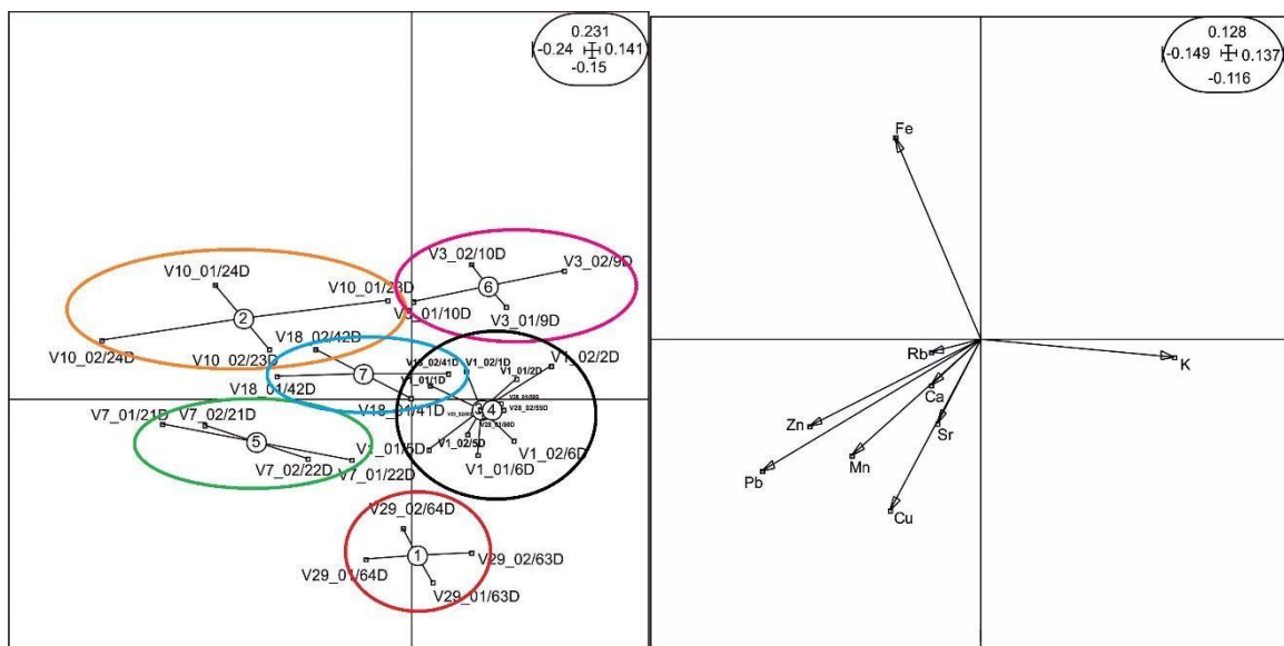
Slika 26. BG-PCA za sortu graševina, svrstana u grupe prema elementnom sastavu K, Ca, Mn, Fe, Cu, Zn, Rb, Sr i Pb. S lijeve strane prikazana je projekcija uzoraka s gravitacijskim centrima grupa (1-Brnjanec, 2-Dabac, 3- Furmek, 4-Horvatić, 5-Katalenić, 6- Piršlin, 7-Stankić). S desne strane je grafički prikaz korelacija varijabli s prve dvije osi koje ujedno objašnjavaju najviše varijance.
