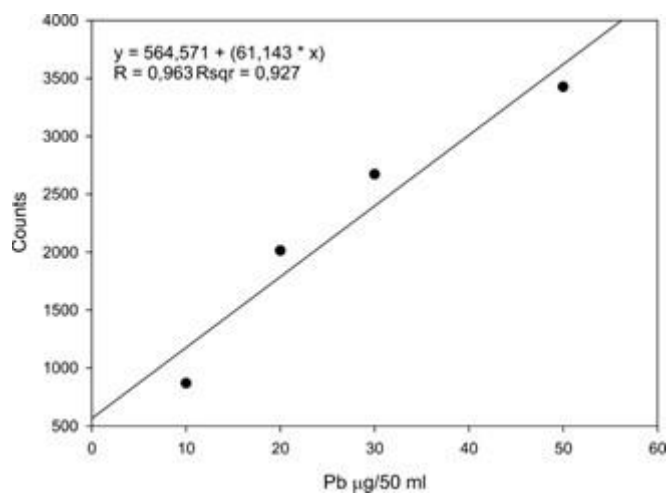
Slika 11. Kalibracijski pravac za element Pb.
