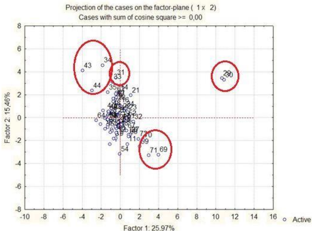
Slika 18. Dijagram faktorskog prikaza za uzorke tla.
