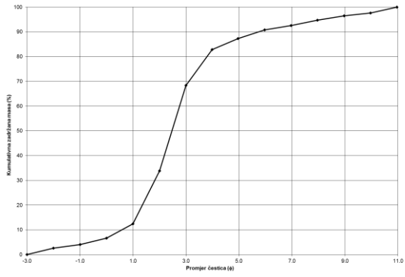
Prilog 19: Kumulativna krivulja uzorka Funtana izvana 2-3
