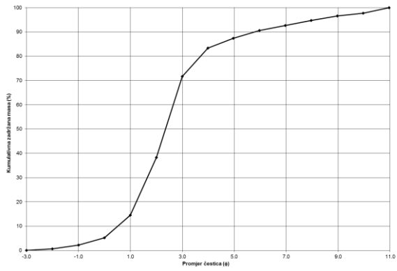
Prilog 21: Kumulativna krivulja uzorka Funtana izvana 4-5
