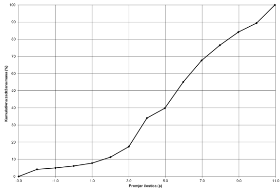
Prilog 25: Kumulativna krivulja uzorka Saline izvana 0-1
