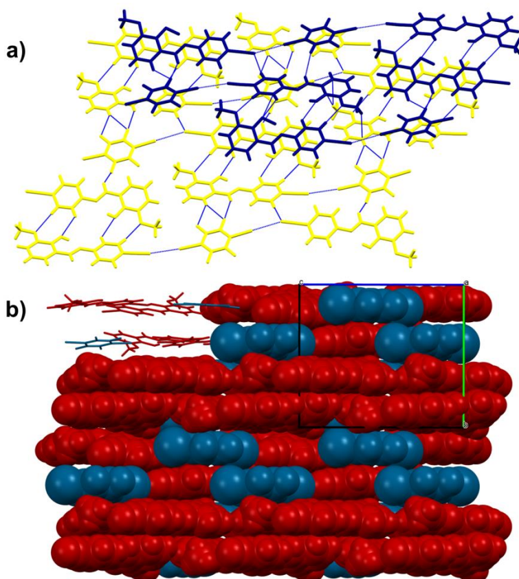
Slika 25. Prikaz: a) povezivanja 2D-mreža kokristala (ov4abn) 2 (pditfb) u 3D-mreže pomoću vodikovih veza. Međumolekulske interakcije prikazane su plavom iscrtkanom linijom i b) dijagram slaganja 3D supramolekulskih mreža pomoću međumolekulskih interakcija.
