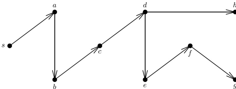
SLIKA B.24. DFS-stablo T_d neusmjerene mreže G .
