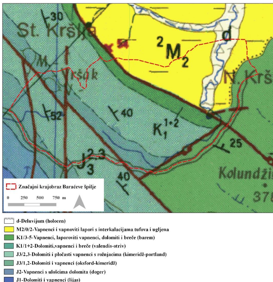
Slika 3. Geološka karta istraživanog područja Baračevih špilja (napravljena prema Polšak i dr., 1976, O GK; List Bihać, izvorno mjerilo 1:100 000)
