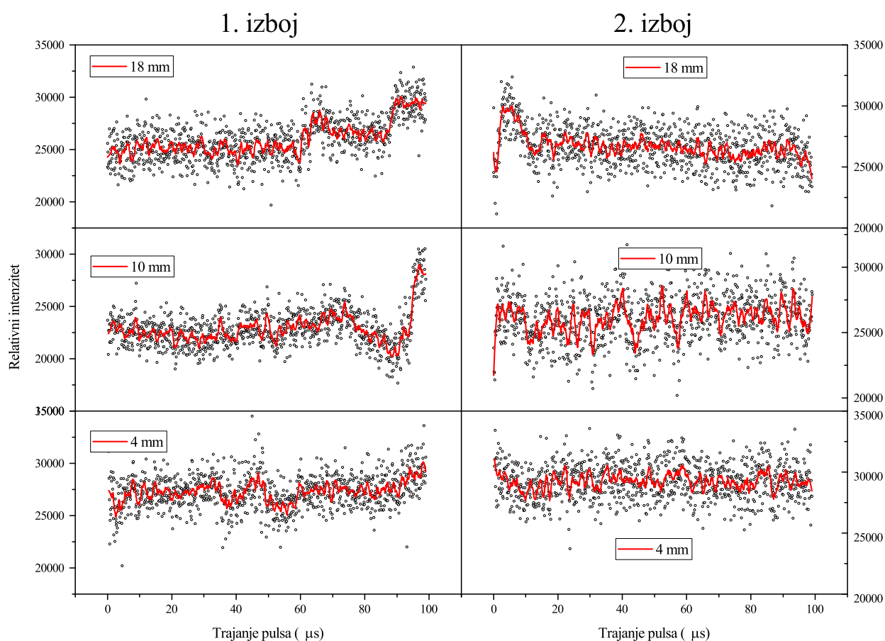
Slika 5.51: Ovisnost emisijskog intenziteta (He 588 nm) o širini naponskog pulsa kad je laserski puls fiksiran u vremenu na primarni izboj (lijevo) i sekundarni izboj (desno) kada je plazmeni mlaz u kontaktu s vodom na udaljenostima od 18, 10 i 4 mm, energija lasera 45 mJ, V=4 kV
