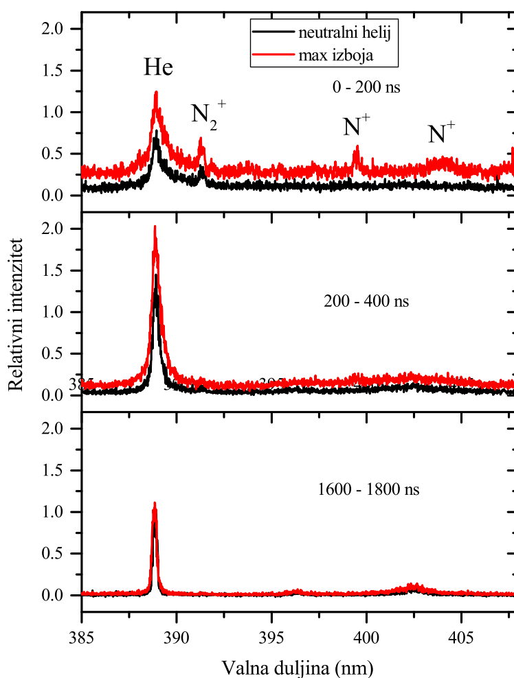
Slika 5.29: Optički emisijski spektar laserski inducirane plazme za različite vremenske prozore
