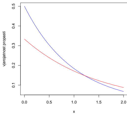
Slika 2.2: Prikaz funkcija \vartheta_3(x) i \vartheta_4(x)
