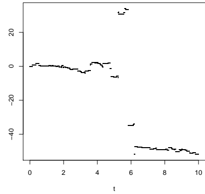
Slika 1.5: 1– stabilan proces
