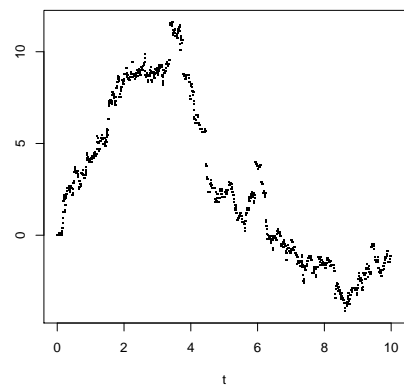
Slika 1.7: 1.8– stabilan proces
