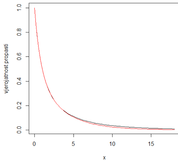
Slika 2.8: Funkcije propasti \vartheta_1(x) (crno) i \vartheta_2(x) (crveno)
