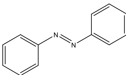
Slika 18. Struktura azobenzena
