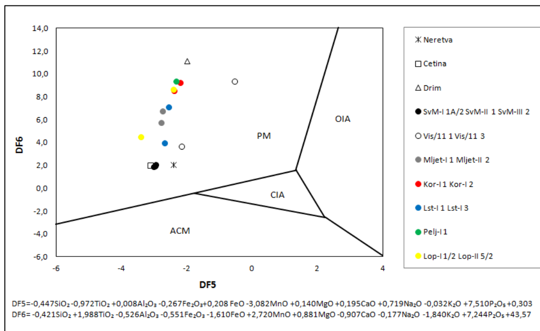
Slika 5.4. Dijagram za određivanje geotektonskog smještaja izvornih predjela pješkovitih sedimenata na osnovu diskriminantnih funkcija baziranih na sadržaju glavnih elemenata primijenjenih na pleistocenske pijeske otoka južnog Jadrana te poluotoka Pelješca i recentne pijeske Neretve, Cetine i Drima (prema Bhatia, 1983). Legenda za skraćenice dana je na Slici 5.3.
