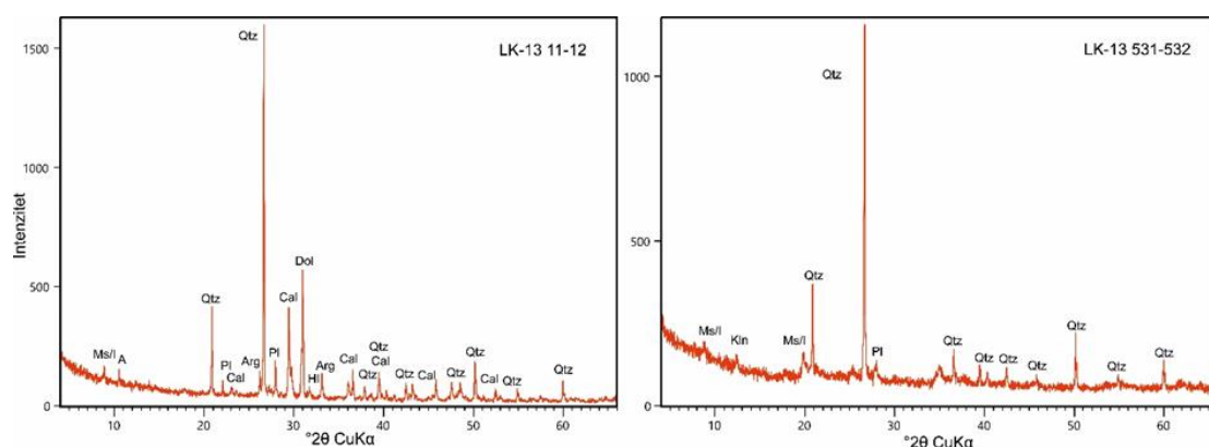
Slika 77: Rendgenogrami uzorka iz jedinice LU-13-1 (11-12 cm) i uzorka iz jedinice LU-13-4 (531-532 cm). Simboli (Kretz, 1983): Cal-kalcit, Hl-halit, Dol-dolomit, Arg-aragonit, Qtz-kvarc, Pl-plagioklas, A-amfibol, Ms/I-muskovit/illit, Kln-kaolinit.
