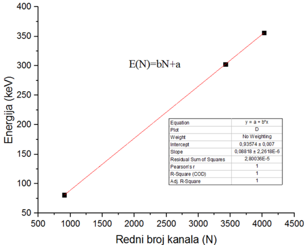
Slika 7.18: Kalibracijska funkcija dobivena linearnog regresijom.
