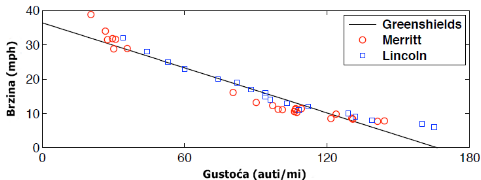
Slika 3.2: Krivulja dobivena Greenshieldsovim zakonom (3.2) za podatke Meritt Parkway i Lincoln Tunnel.
