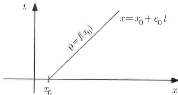
Slika 5.4: Metoda karakteristika za određivanje krivulja x = X(t) duž kojih je rješenje od (5.1) konstantno.
