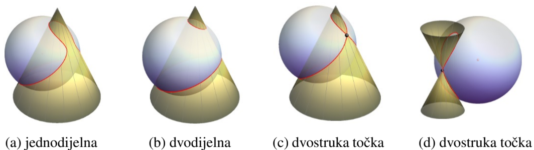
Slika 3.50: Prave prostorne krivulje kod prodora sfere i stošca Izvor:[8]
