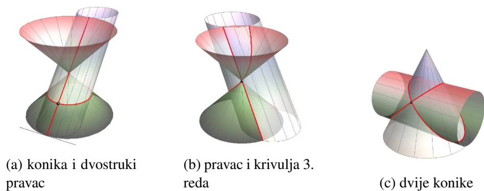
Slika 3.30: Raspadnute prostorne krivulje kod prodora stošca i valjka Izvor:[8]
