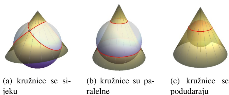
Slika 3.51: Raspadnute prostorne krivulje kod prodora sfere i stošca - kružnice Izvor:[8]
