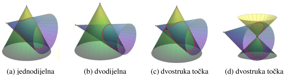
Slika 3.16: Prave prostorne krivulje kod prodora dvaju stožaca
