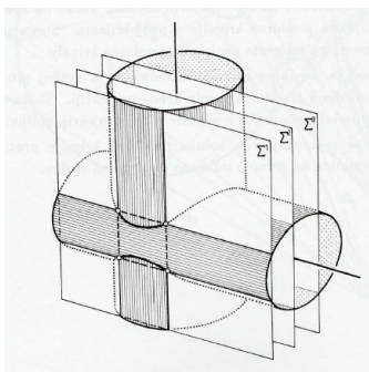
Slika 3.1: Pomoćne ravnine kod prodora dvaju valjaka
