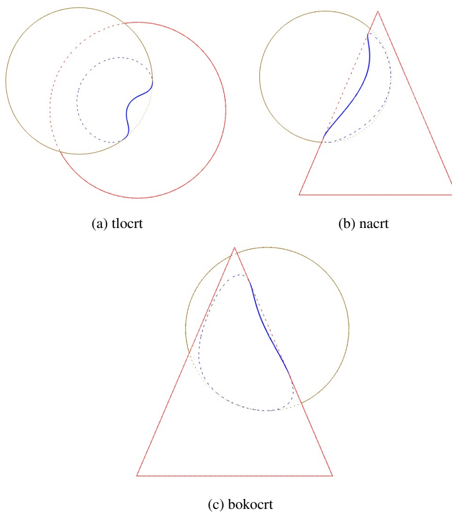
Slika 3.54: Ortogonalne projekcije stošca, sfere i njihove prodorne krivulje - Rhinoceros
