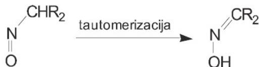
Shema 3. Pregradnja nitrozo spojeva u oksime.
