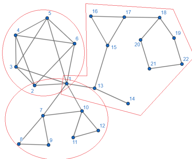
Slika 3.4: Graf G
