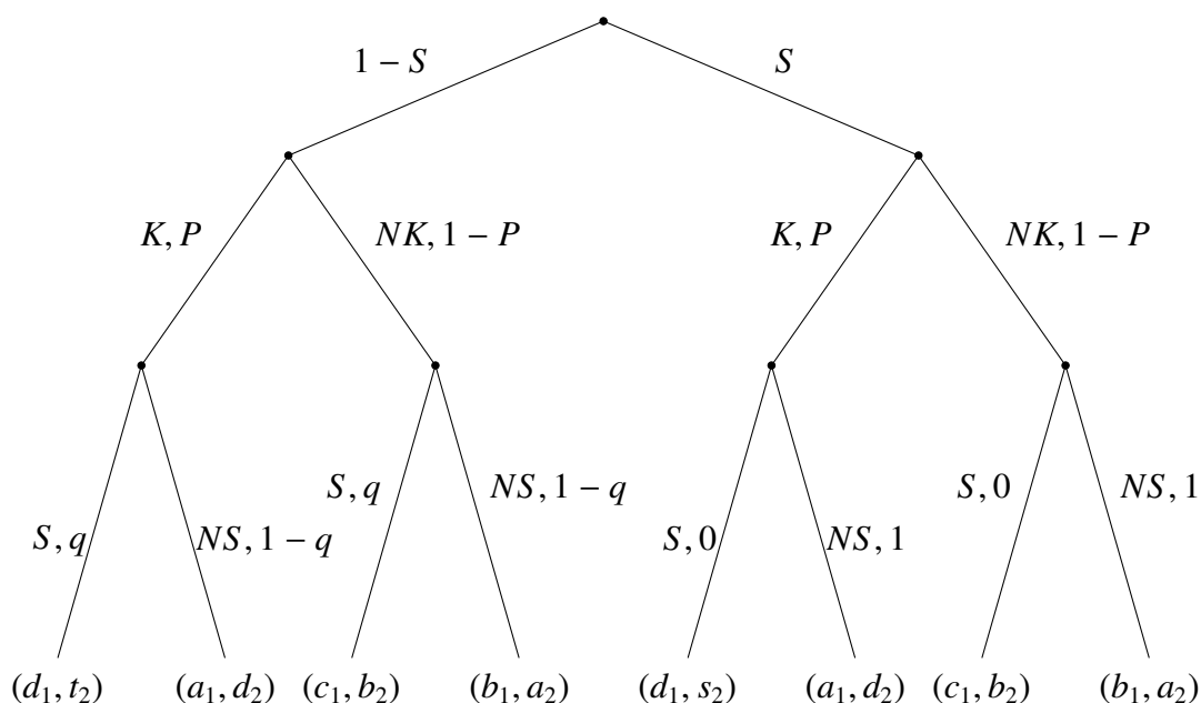
Slika 3.1: Stablo 2
