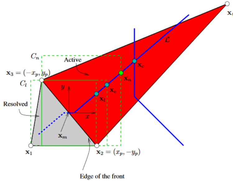
Slika 8. Ubacivanje optimalnog trokuta u mrežu frontal-Delanaury pristupom
