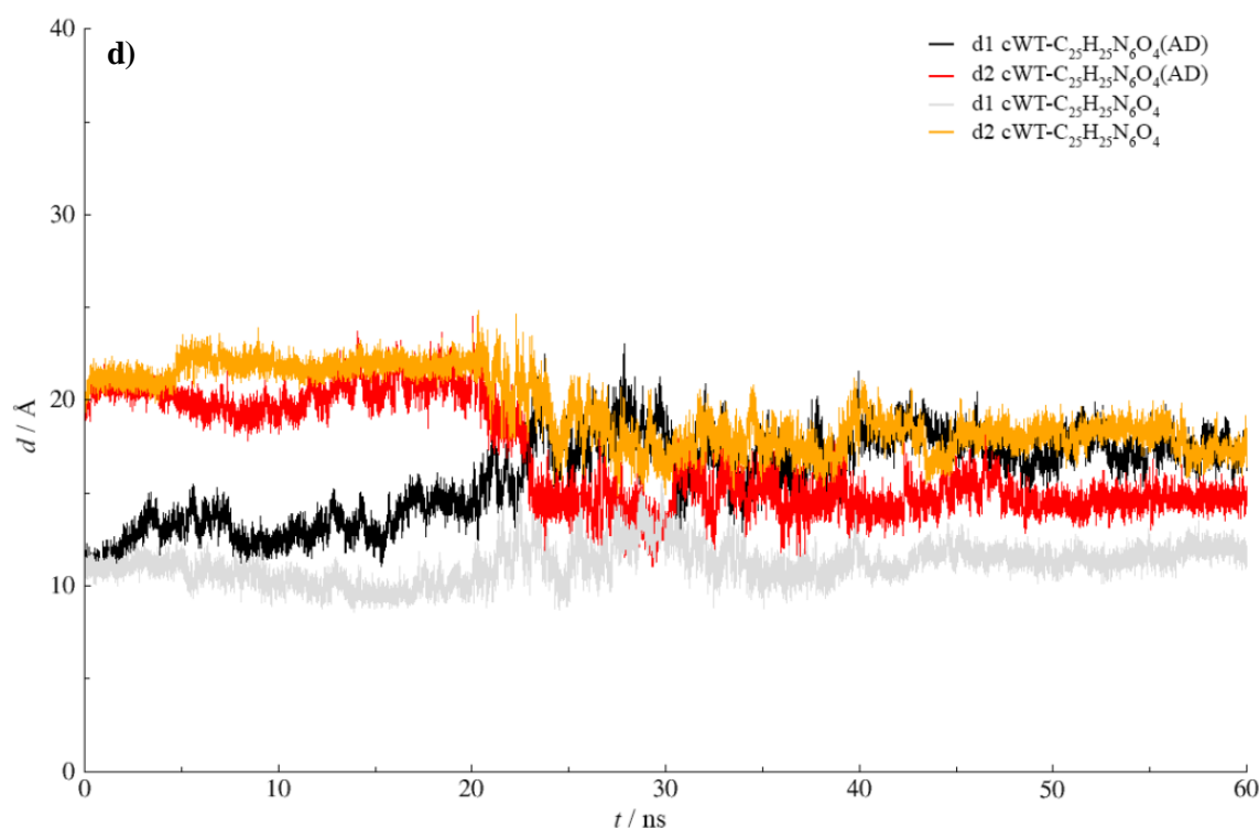
Slika 6. Udaljenosti između Ca atoma aminokiselinskih parova D186-S500 (d1) i Q400-S500 (d2) tijekom MD simulacija. a) Kompleks manje kompaktne DPP III s ligandom 1 dobiven u AUTODOCK-u, cWT_{MD-1}(AD1) i cWT_{MD-1}(AD2) ; b) kompleks kompaktne DPP III s ligandom 1, cWT-1 , c) kompleksi manje kompaktne DPP III s ligandom 2, cWT_{MD-2}(AD) i cWT_{MD-2} , d) kompleksi kompaktne DPP III s ligandom 2, cWT-2(AD) i cWT-2 .
