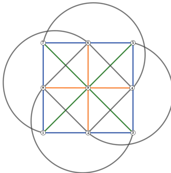
Slika 1.2: 2-(9, 3, 1) dizajn
