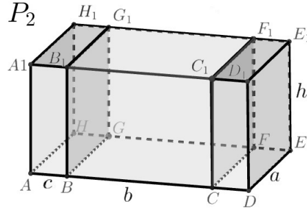
Slika 1.12: Poliedar P_2
