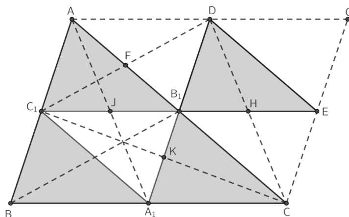
Slika 1.8: p(C_1CD) = \frac{3}{4}p(ABC)
