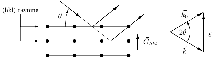
Slika 1.17: Prikaz kristalnih ravnina, upadnog i raspršenog zračenja, i vektora raspršenja.
