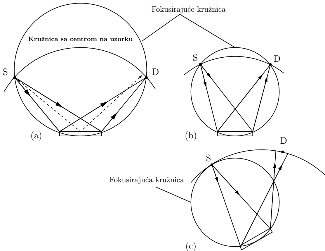
Slika 2.6: Bragg Brentano geometrija.
