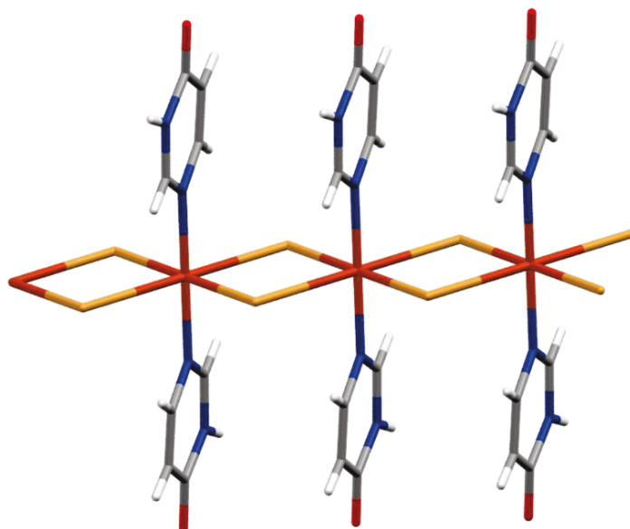
Slika 27. Jednodimenzijnski polimerni lanac koordinacijskog spoja [\text{CuBr}_2(4\text{-pym})_2]_n ( 2 )
