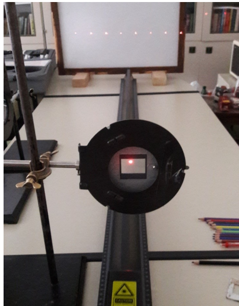
Slika 5.5: Postav za optičku rešetku od 80 zarez/mm
