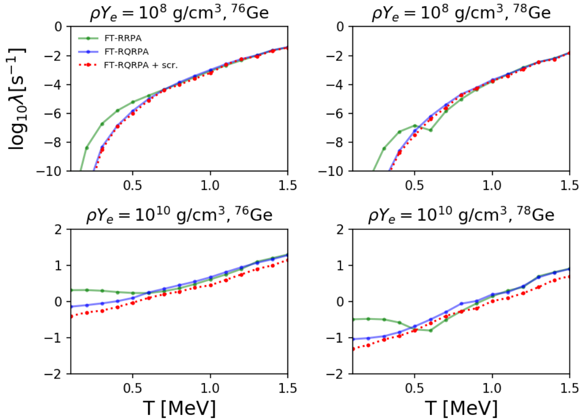
Slika 6.18: Ovisnost logaritma stopa uhvata elektrona o temperaturi za jezgre 76 Ge i 78 Ge, pri gustoćama 10^8 g/cm 3 i 10^{10} g/cm 3 . U izračun su uključeni multipoli J^\pi = 0^\pm, 1^\pm, 2^\pm .
