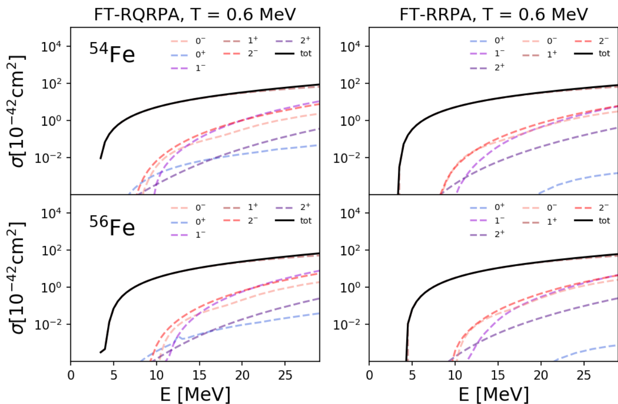
Slika 6.8: Udarni presjek za uhvat elektrona za multipole J^\pi = 0^\pm, 1^\pm, 2^\pm , na jezgrama ^{54}\text{Fe} i ^{56}\text{Fe} pri temperaturi T = 0.6 MeV. Lijevo se nalaze udarni presjeci po multipolima izračunati uz FT-RQRPA račun, a desno FT-RRPA. Temperatura je ispod temperature faznog prijelaza pa korelacije sparivanja imaju značajnu ulogu. Posebno uočavamo multipol 0^+ koji u FT-RRPA računu ima najmanju ulogu, a kod FT-RQRPA računa njegova amplituda je porasla, te ga koristimo kao ilustrativan primjer utjecaja korelacija sparivanja (za više pojediniosti pogledati u tekstu).
