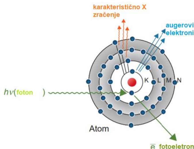
Slika 2.9 Fotoelektrični učinak i procesi koji mogu slijediti [3]
