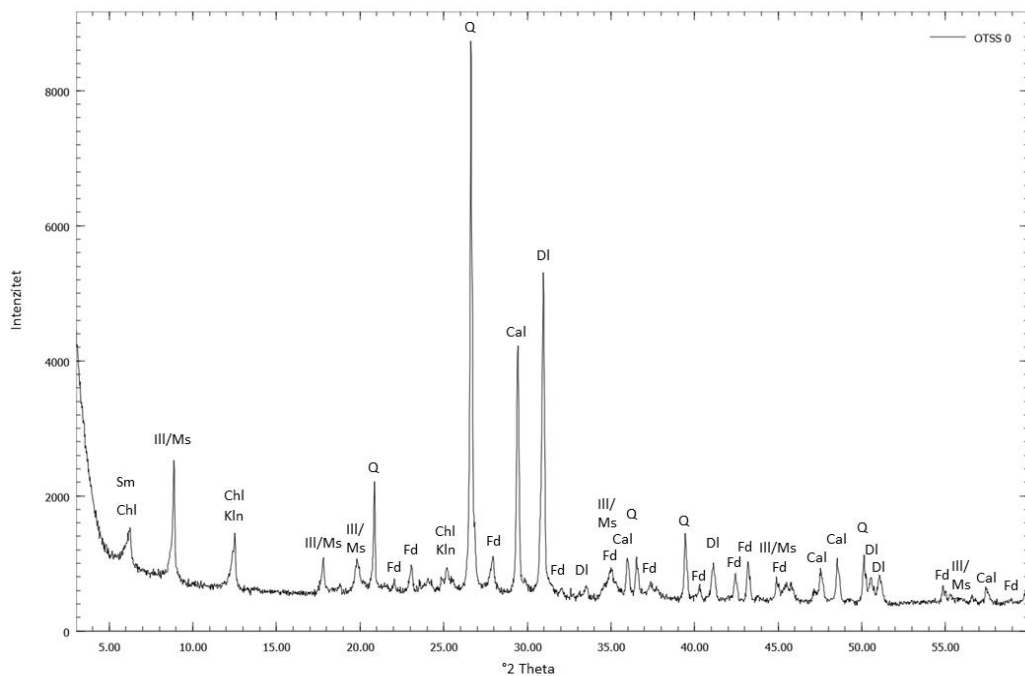
Slika 27. Rendgenska difrakcijska slika sitnozrnatog sedimenta (S20) (Chl – klorit, Sm – smektit, Ill/Ms – illit/muskovit, Kln – kaolinit, Q – kvarc, Fd – feldspat, Cal – kalcit, DI – dolomit)
