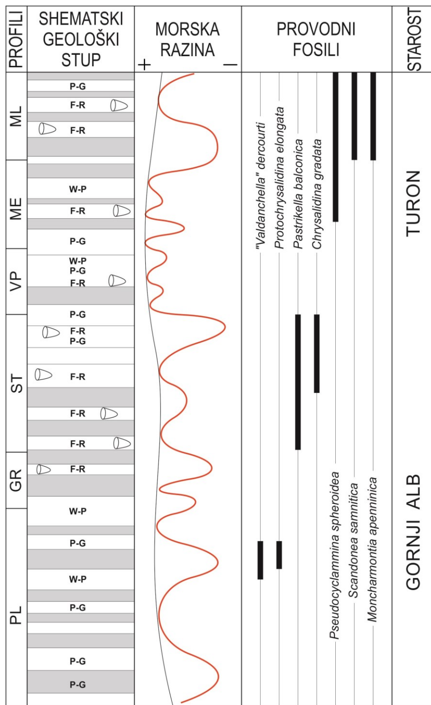
Slika 26. Shematski geološki stup analiziranih profila s relativnom promjenom razine mora (Haq, 2014), starosti i provodnim fosilima.
