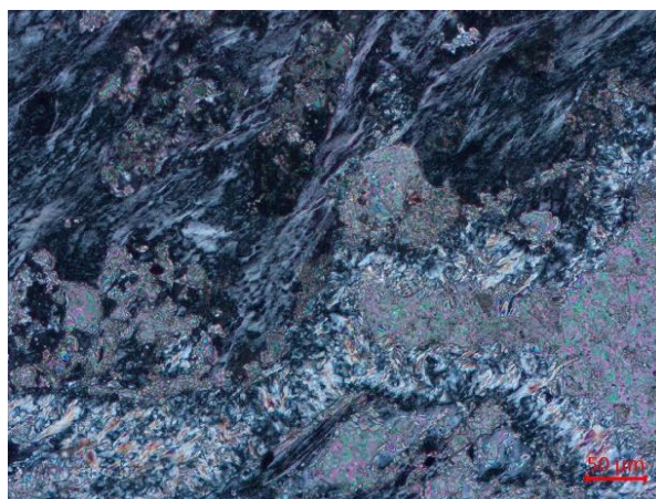
Slika 7.3: Mikrofotografija kalcitne mandule uzorka u1 . Slika napravljena s uključenim analizatorom (N+). Na kontaktu osnove i mandule iskristalizirao je listićavi mineral koji interferira u žutoj boji I.reda (filosilikat?) Crvena linija označava 50 \mu\text{m} .
