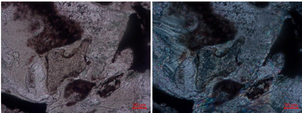
Slika 7.20: Mikrofotografije uzorka u5 . Lijevo (N-), desno (N+). Fragment vulkanskog stakla („glass shard“). Crvena linija označava 50 µm.
