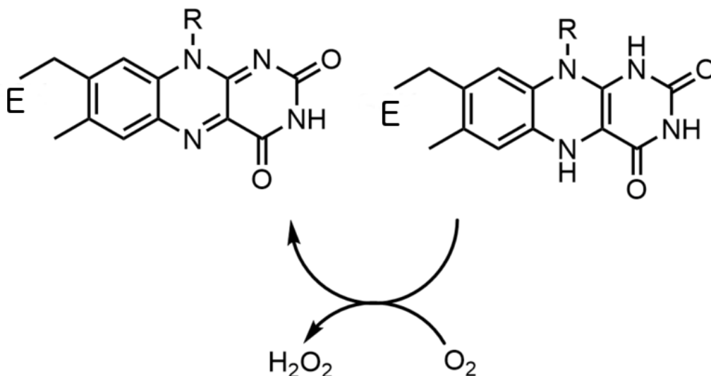
Slika 2. Oksidacija reduciranog kofaktora FADH 2 do oksidiranog kofaktora FAD uz pomoć supstrata kisika. Konačni produkt reakcije oksidacije FADH 2 kisikom jest vodikov peroksid.
