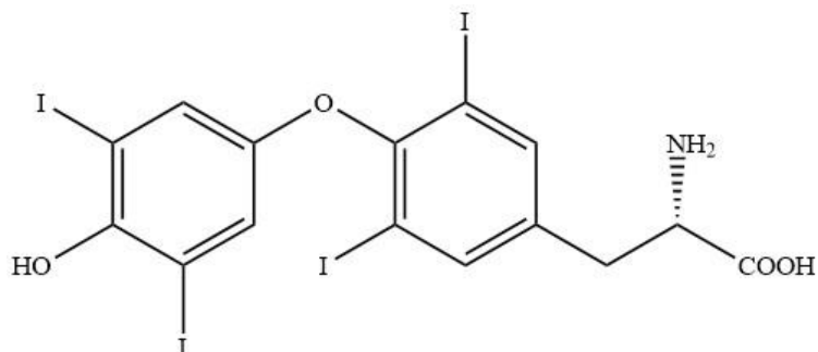
Slika 1. Levotiroksin, T 4 .
