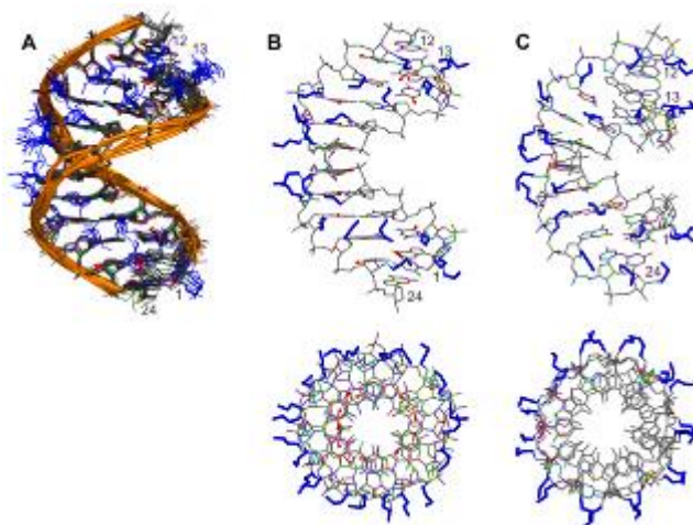
Slika 4.5. (A) superpozicija devet struktura dvolančane 2'-MOE RNA metilirane na ugljikovom atomu u položaju 5 (B) struktura dvolančane 2'-MOE RNA metilirane na ugljikovom atomu u položaju 5 (C) nemetilirana dvolančana 2'-MOE RNA
