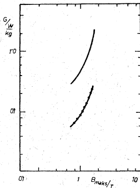
Sl. 4. Usporedba gubitaka u jezgri ( G ) za konvencionalnu Fe_3\%Si slitinu (puna linija), amornu slitinu Fe_{82}B_{10}Si_8 (kružići) iste debljine pri sinusnoj indukciji magnetskog polja B frekvencije 60 Hz
